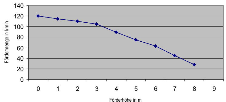
Förderkurve WATERSAN +
