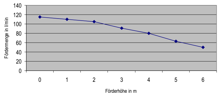
Förderkurve WATERSAN 6
