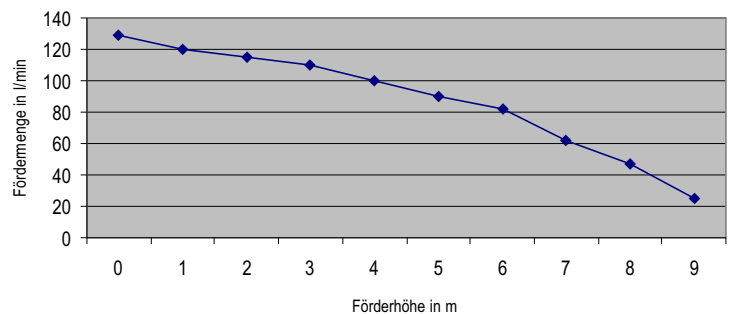
Förderkurve WATERSAN 4
