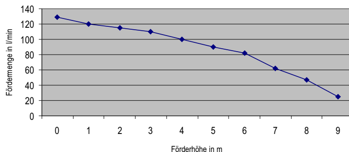
Förderkurve WATERSAN 4
